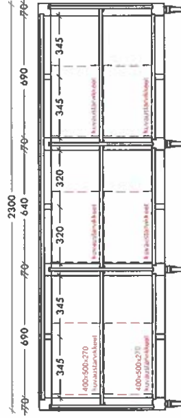
PYSTYLEIKKAUS 1:20
