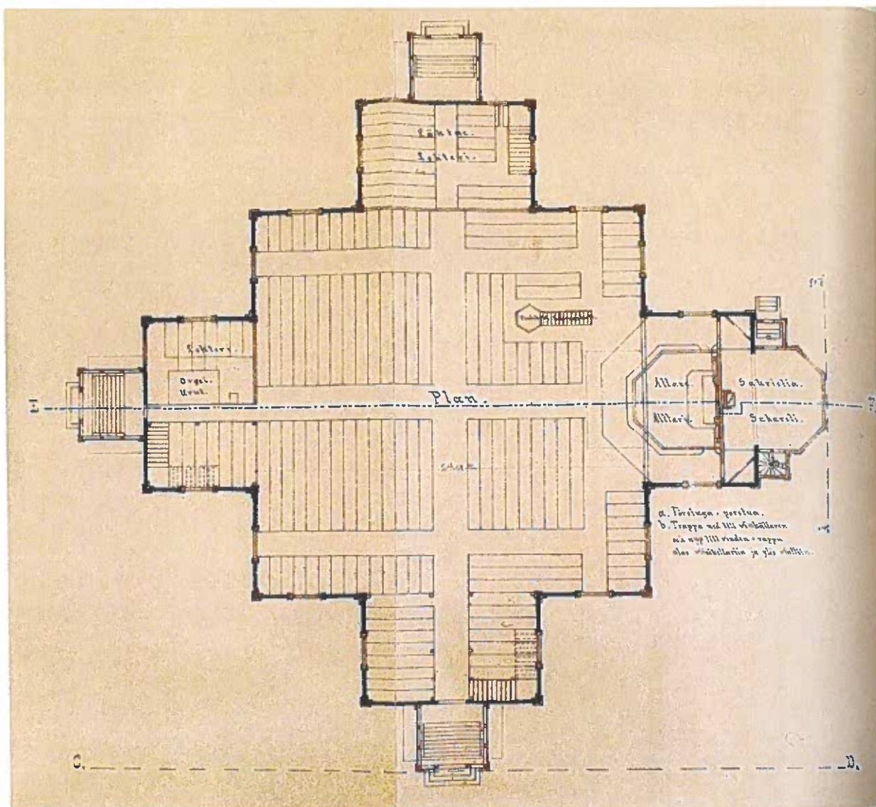
Kuva: Alfred Cavénin Kangasniemen kirkon pohjapiirustus vuodelta 1889. Keisarillisen senaatin talousosaston hyväksymä ja noudatettavaksi vahvistama 9.5.1890. Piirustuksessa on esitetty yläosassa parvikerrokset ja alaosassa pohjakerros. Suunnitelma on todennäköisesti toteutunut pitkälti esitetyn kaltaisena. Kangasniemen seurakunnan kuvapankki.
