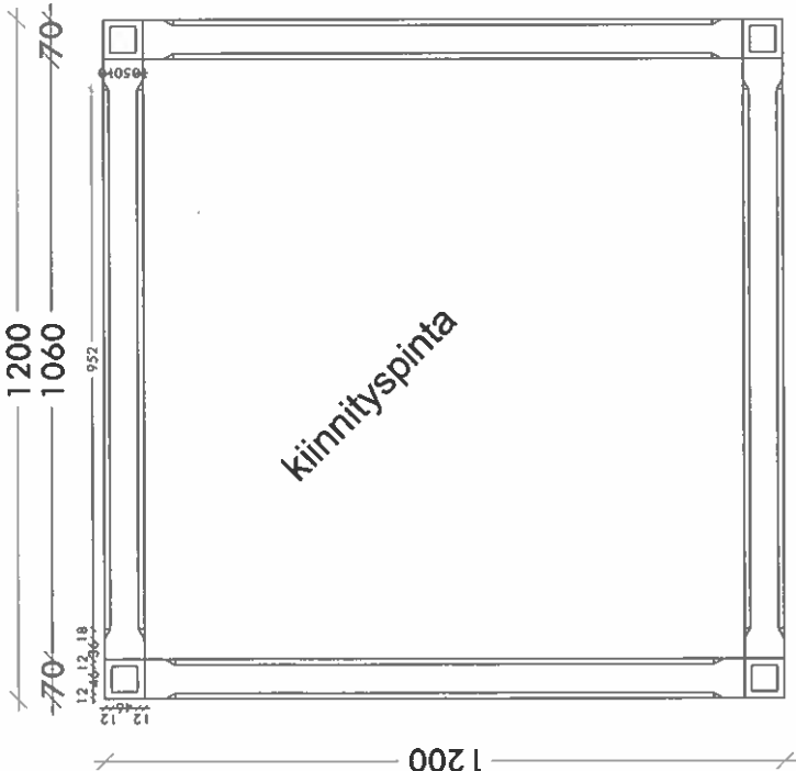
PROJEKTIO EDESTÄ 1:10
