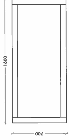
PROJEKTIO PÄÄLTÄ
