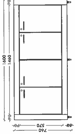
PROJEKTIO EDESTÄ 1:20
