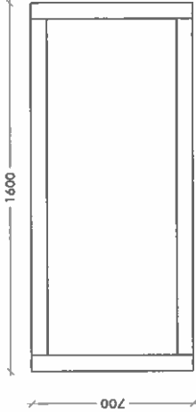
PROJEKTIO PÄÄLTÄ 1:20
