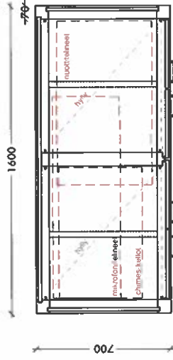
VAAKALEIKKAUS
