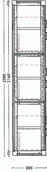
VAAKALEIKKAUS
