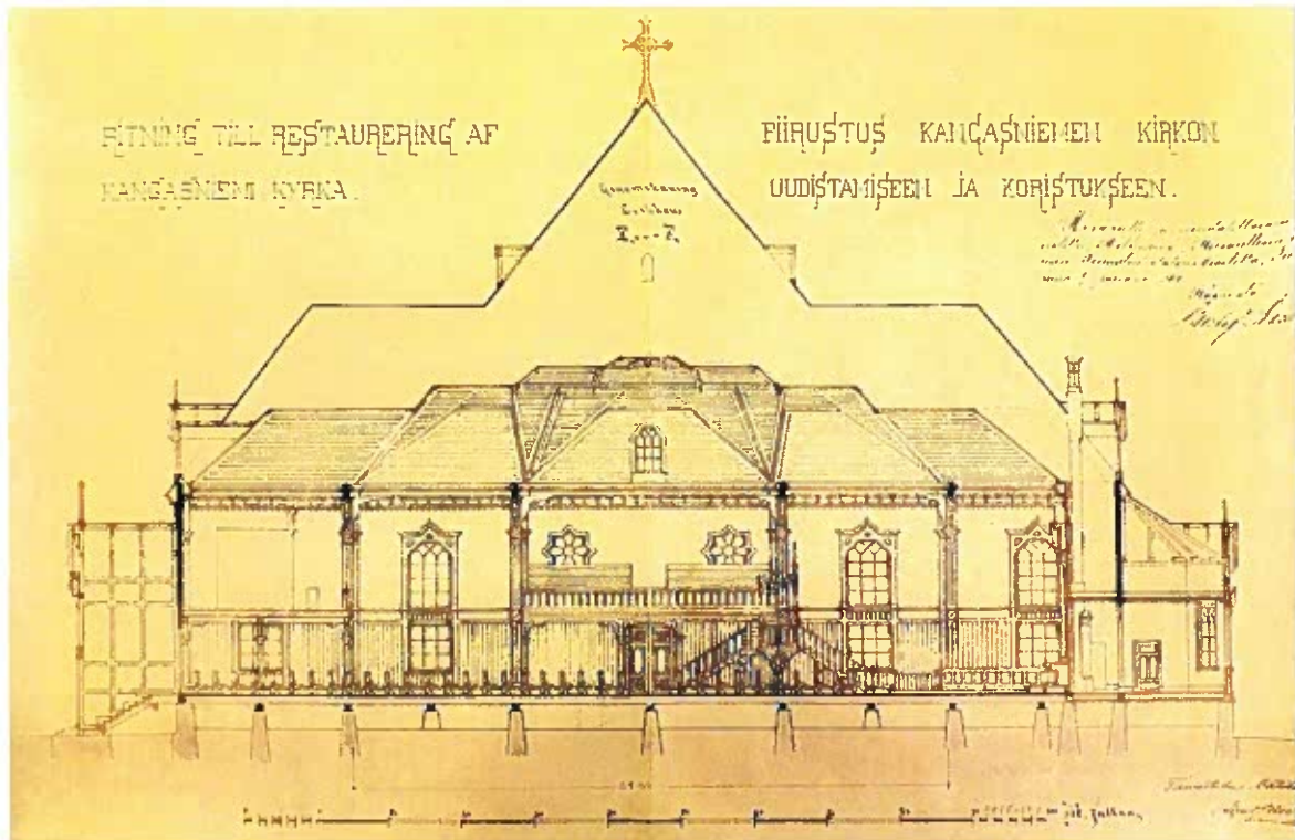
Kuva: Alfred Cavénin leikkauspiirustuksesta näkyy hyvin kirkon sisätilojen uudet koristeelliset lisätoitukset ja konsolit. Keisarillisen senaatin talousosaston hyväksymä ja noudatettavaksi vahvistama 9.5.1890. Kangasniemen seurakunnan kuvapankki.
