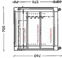
PYSTYLEIKKAUS 1:20
