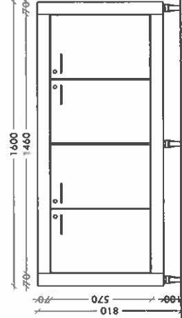
PROJEKTIO EDESTÄ 1:20
