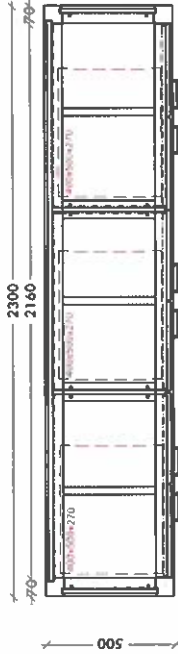
VAAKALEIKKAUS 1:20
