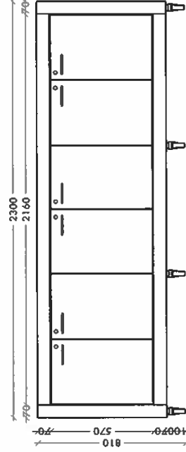
PROJEKTIO EDESTÄ 1:20
