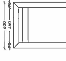
SIVUPROJEKTIO 1:20
