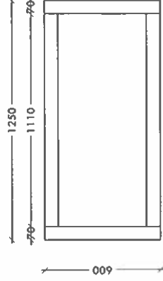
PROJEKTIO PÄÄLTÄ
