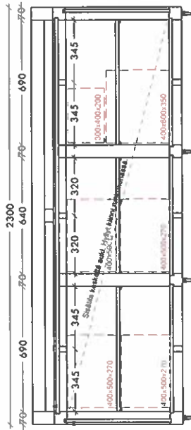
PYSTYLEIKKAUS 1:20
