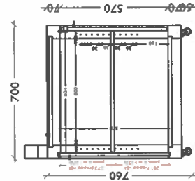
PYSTYLEIKKAUS
